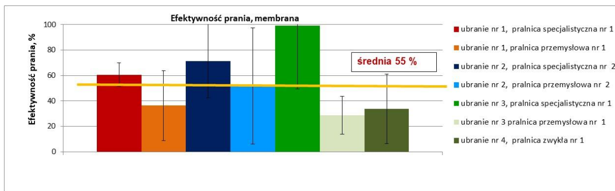
Rysunek 6. Efektywność procesu prania w odniesieniu do membrany stosowanej w odzieży ochronnej dla strażaka użytkowanej jednorazowo w komorze ćwiczeń lub podczas działań ratowniczo-
