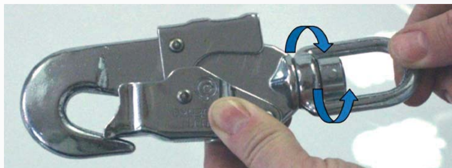
Rys. 6. Sprawdzenie możliwości ruchu elementu obrotowego zatrzaskownika [3] Fig. 6. Rotation test of a swivel element of the connector [3]
