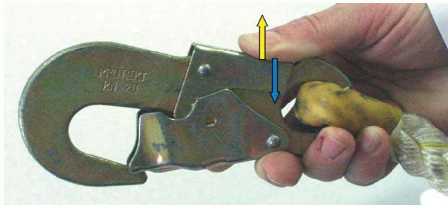
Rys. 5. Sprawdzenie samoczynnego blokowania się zatrzaskownika [3] ← – kierunek dociśnięcia dźwigni blokady → – kierunek samoczynnej, prawidłowej reakcji dźwigni blokady
