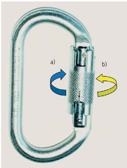
Rys. 4. Sprawdzenie zatrzaskownika z tulejką samoczynnie powracającą do pozycji zablokowanej [3] a) – kierunek ręcznego odblokowania tulejki b) – kierunek automatycznego powrotu tulejki do stanu zablokowania
