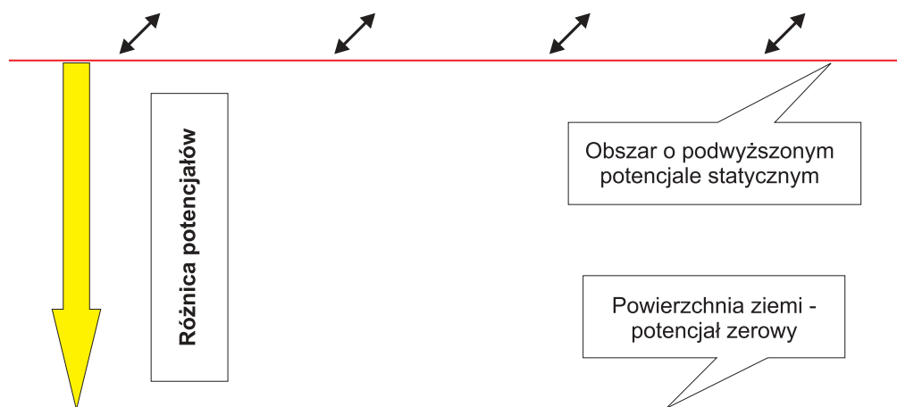
Rys. 2. Mechanizm powstawania wyładowań atmosferycznych.
