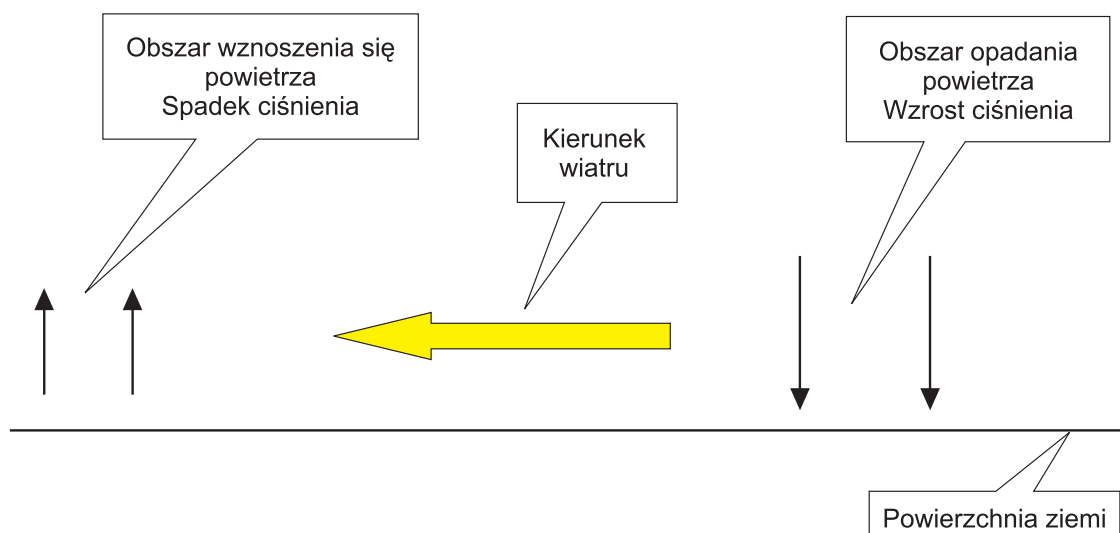
Rys.1. Mechanizm powstawania wiatru
