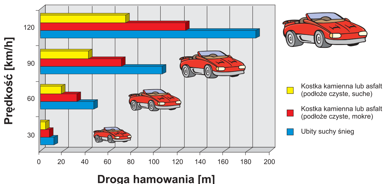
WYKRES – Droga hamowania pojazdu samochodowego w zależności od jego prędkości i rodzaju nawierzchni.
