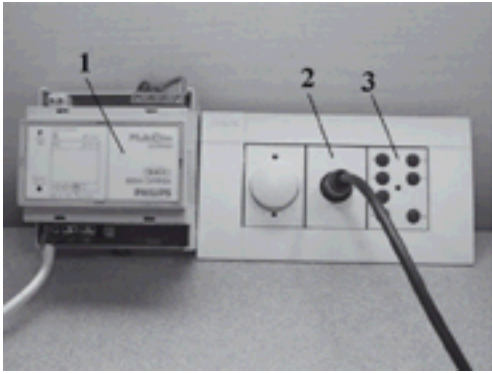
Rys. 1. Elementy sterujące systemu: 1 – moduł sterujący; 2 – interfejs umożliwiający komunikację użytkownika z systemem; 3 – panel sterujący z wbudowanym czujnikiem podczerwieni
