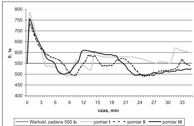
Rys. 7. Zmiany poziomu natężenia oświetlenia przy włączonej opcji utrzymania stałego poziomu natężenia oświetlenia, po odsłonięciu okien
