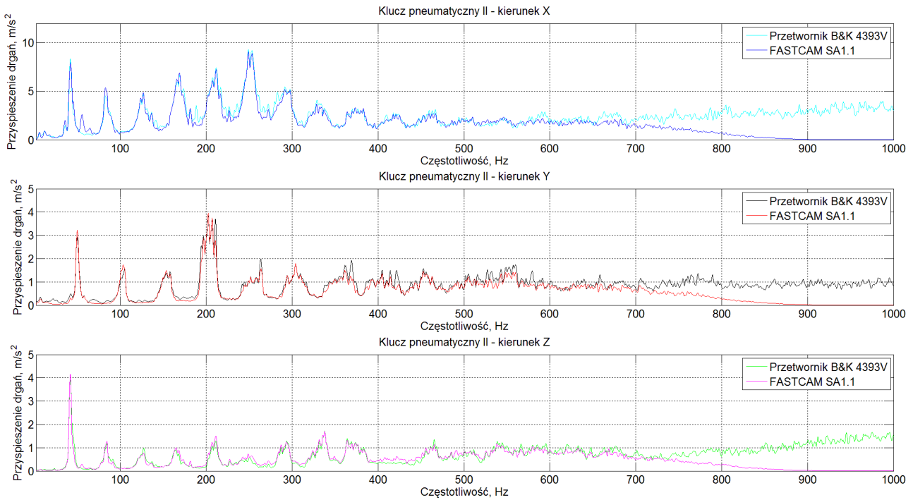
Rys. 2. Przykładowe widma przyspieszeń drgań uzyskane na podstawie analizy obrazu ruchu oscylacyjnego i przy wykorzystaniu klasycznego układu pomiarowego [źródło: rys. powstał przy wykorzystaniu środowiska MATLAB]
