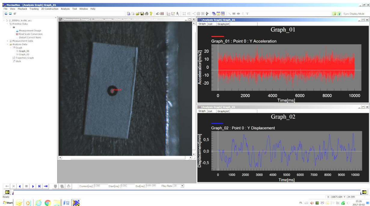
Fot. 4. Przykładowe okno oprogramowania podczas wyznaczania przebiegów czasowych przemieszczenia i przyspieszenia drgań [źródło: fot. powstała przy wykorzystaniu oprogramowania MoviasNeo 2D v. 2.54.]
