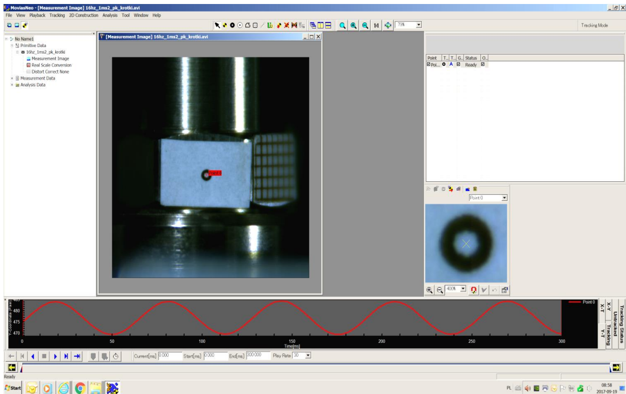
Fot. 3. Przykładowe okno oprogramowania podczas śledzenia punktu pomiarowego [źródło: fot. powstała przy wykorzystaniu oprogramowania MoviasNeo 2D v. 2.54.]
